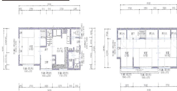
1階 平面図
